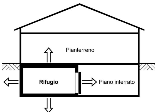
Figura 2.1 Deflusso di calore dal rifugio di un edificio non sufficientemente isolato secondo gli standard odierni (rappresentazione schematica)
