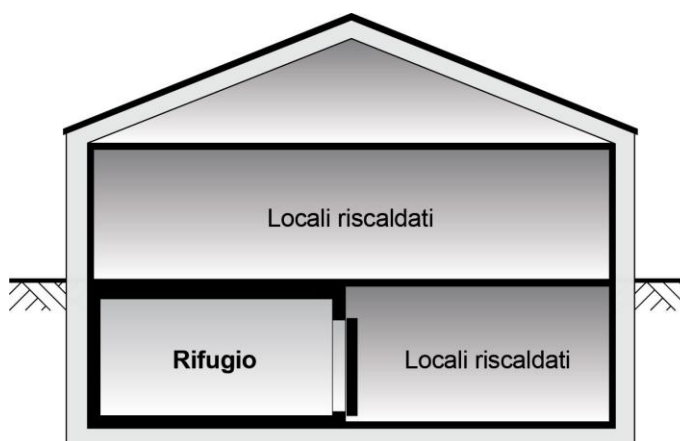
Figura 4.2 Perimetro isolato chiuso nel caso di locali con riscaldamento attivo o passivo al piano interrato
