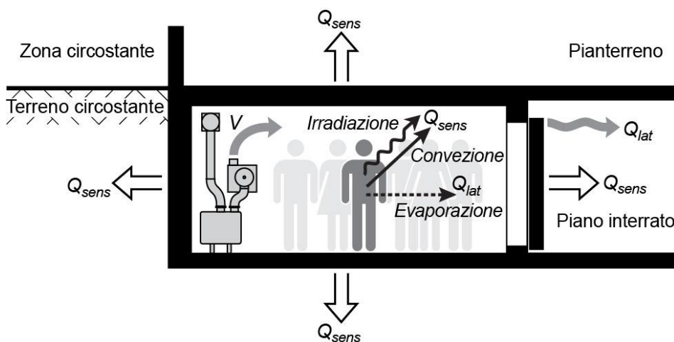
Figura 3.1 Calore ceduto dagli occupanti ed evacuazione del calore dal rifugio
