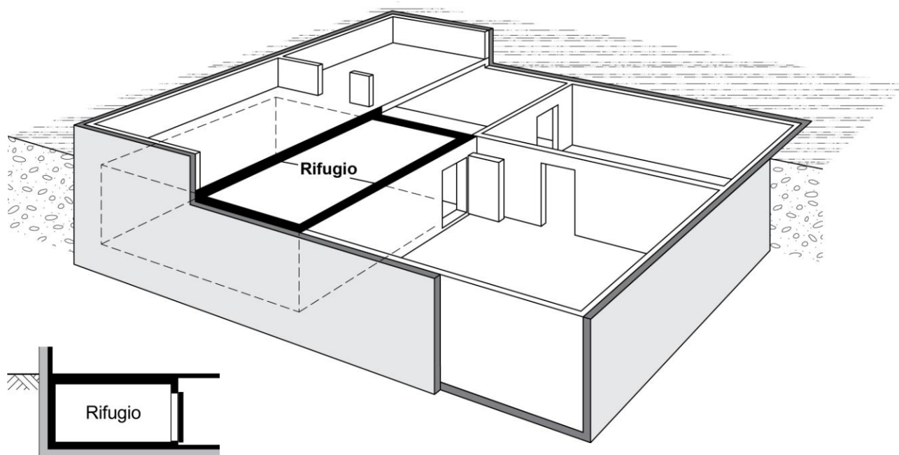
Figura 4.7 Isolamento integrale dell'edificio e dei piani interrati, rifugio compreso
