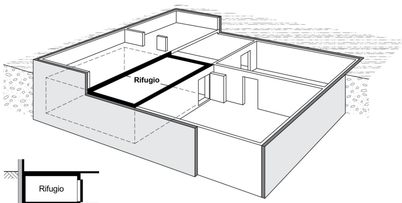
Figura 4.5 Isolamento perimetrale delle pareti a contatto con il terreno e su tutta la loro altezza
