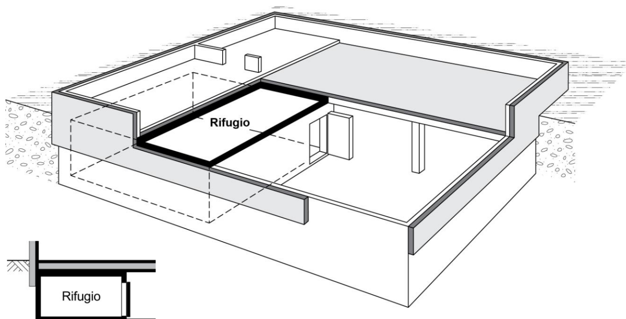
Figura 4.6 Isolamento di tutta la soletta del piano interrato
