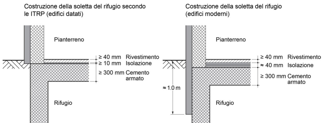
Figura 2.4 Isolazione della soletta del rifugio secondo le ITRP e isolamento degli edifici costruiti secondo gli standard moderni
