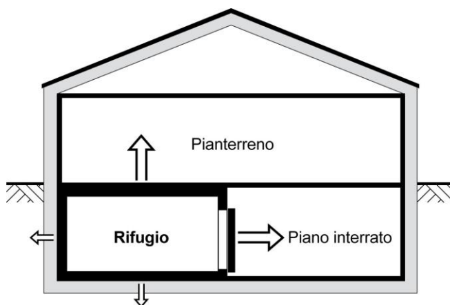
Figura 2.3 Deflusso di calore dal rifugio situato all'interno del perimetro isolato (rappresentazione schematica)
