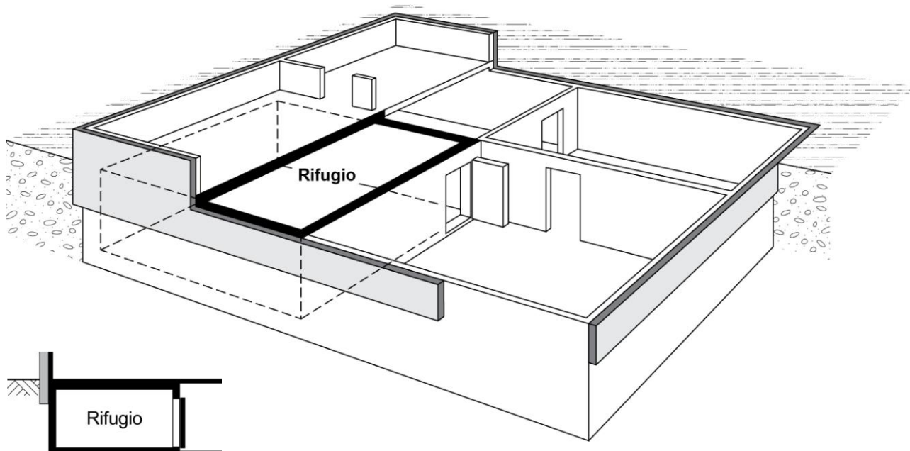
Figura 4.3 Isolamento perimetrale delle pareti interrate fino alla profondità di penetrazione del gelo
