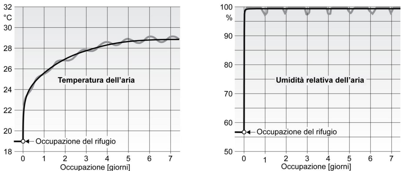
Figura 3.3 Andamento tipico della temperatura e dell'umidità relativa dell'aria interne in caso d'occupazione del rifugio (rappresentazione schematica)
