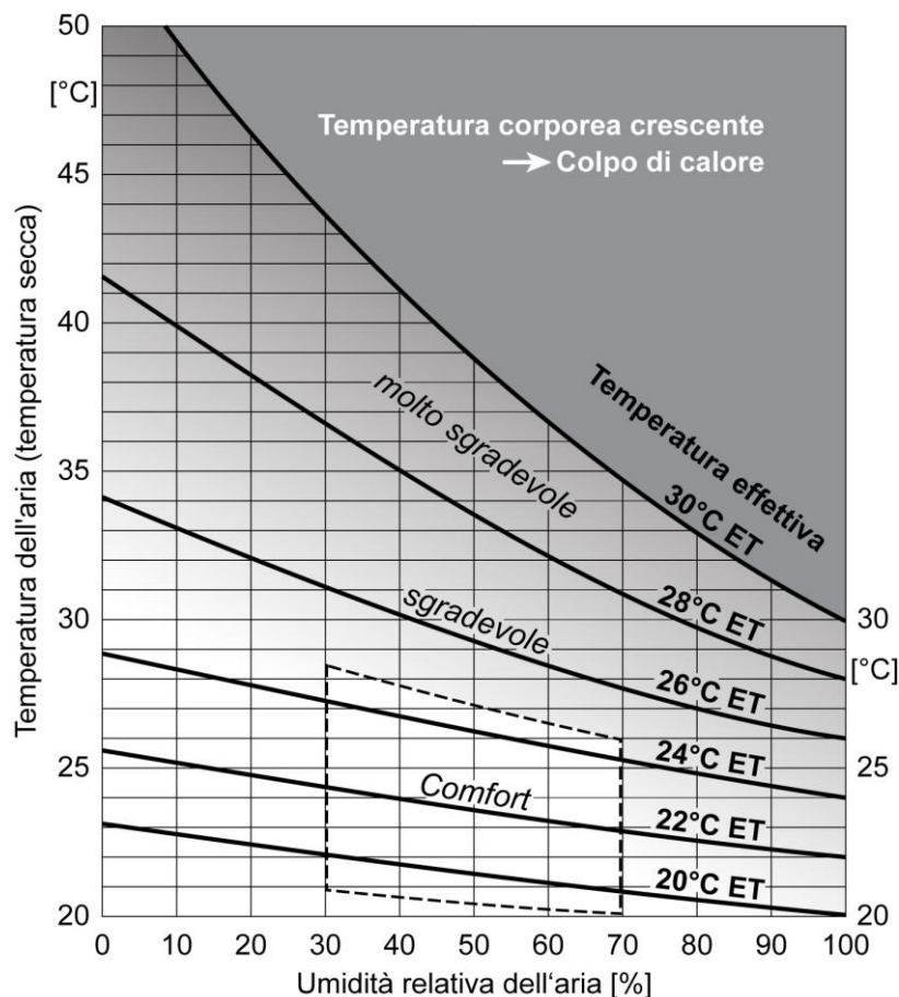
Figura 3.4 Temperatura effettiva ( T_{eff} ) con una velocità dell'aria di 0,1 m/s e percezione delle condizioni climatiche, nonché limite climatico fisiologico dell'essere umano
