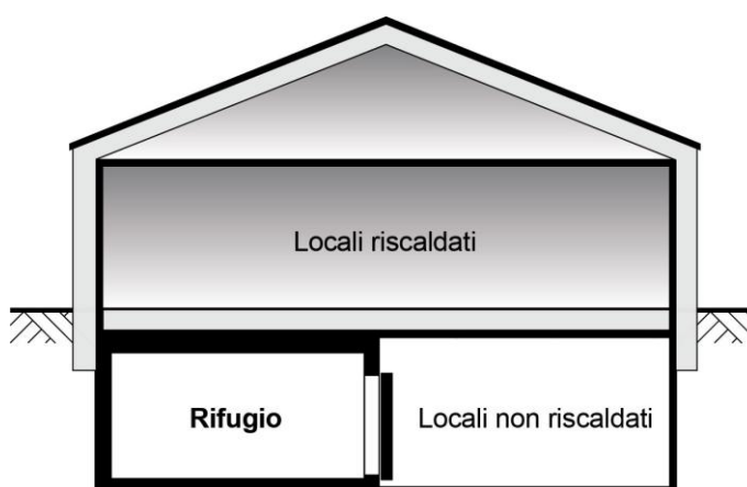
Figura 4.1 Perimetro isolato chiuso e isolamento perimetrale nel caso di locali non riscaldati al piano interrato
