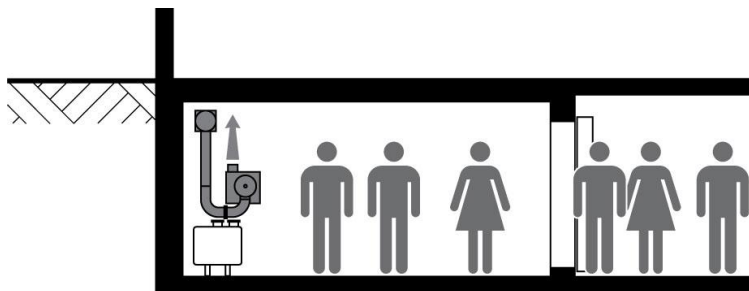
Figura 5.1 Funzionamento senza filtri antigas (FSF) e occupazione a rotazione
