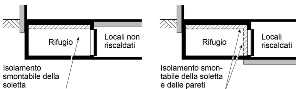
Figura 4.4 Concetto d'isolamento termico con isolamento perimetrale e isolamento smontabile nel rifugio
