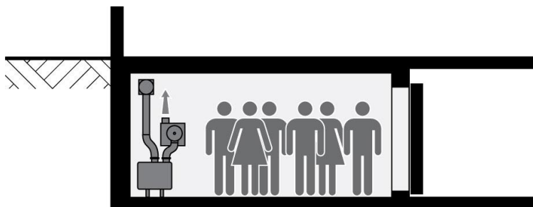
Figura 5.2 Funzionamento con filtri antigas e occupazione autarchica
