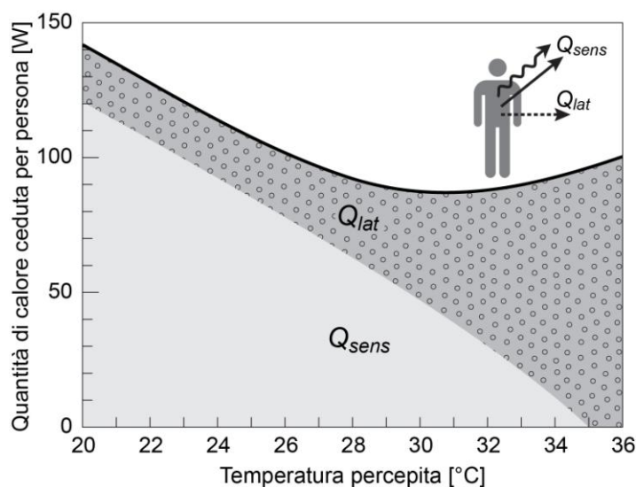
Figura 3.2 Quantità di calore secco (sensibile) e umido (latente) in funzione della temperatura ceduta dall'essere umano all'ambiente circostante
