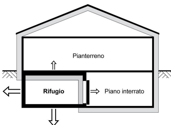
Figura 2.2 Deflusso di calore dal rifugio situato all'esterno del perimetro isolato (rappresentazione schematica)
