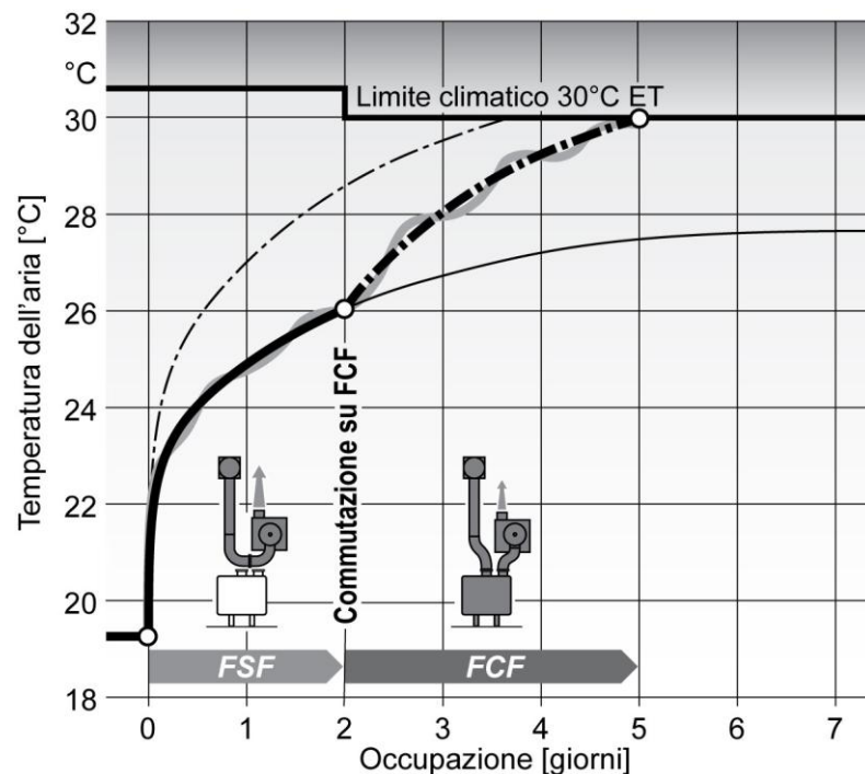
Figura 5.3 Aumento della temperatura nel rifugio, prima con funzionamento senza filtri antigas (FSF) e occupazione a rotazione, poi commutazione sul funzionamento con filtri antigas (FCF) e un'occupazione autarchica (rappresentazione schematica)
