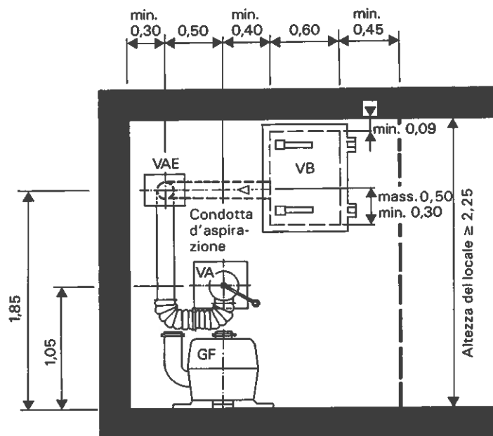
Prospetto Sistemazione con coperchio blindato alto (p. es. in caso di falda freatica e nei locali alti)
