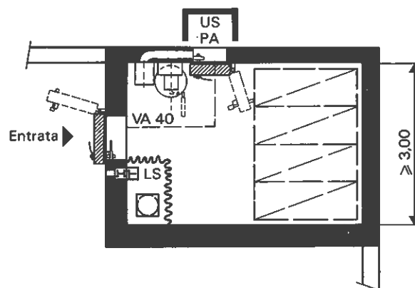
Figura 2.4-6 Pianta per 12 posti protetti (superficie \geq 13 m 2 )
