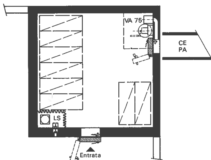
Figura 2.4-10 Pianta per 24 posti protetti (superficie \geq 25 \text{ m}^2 )
