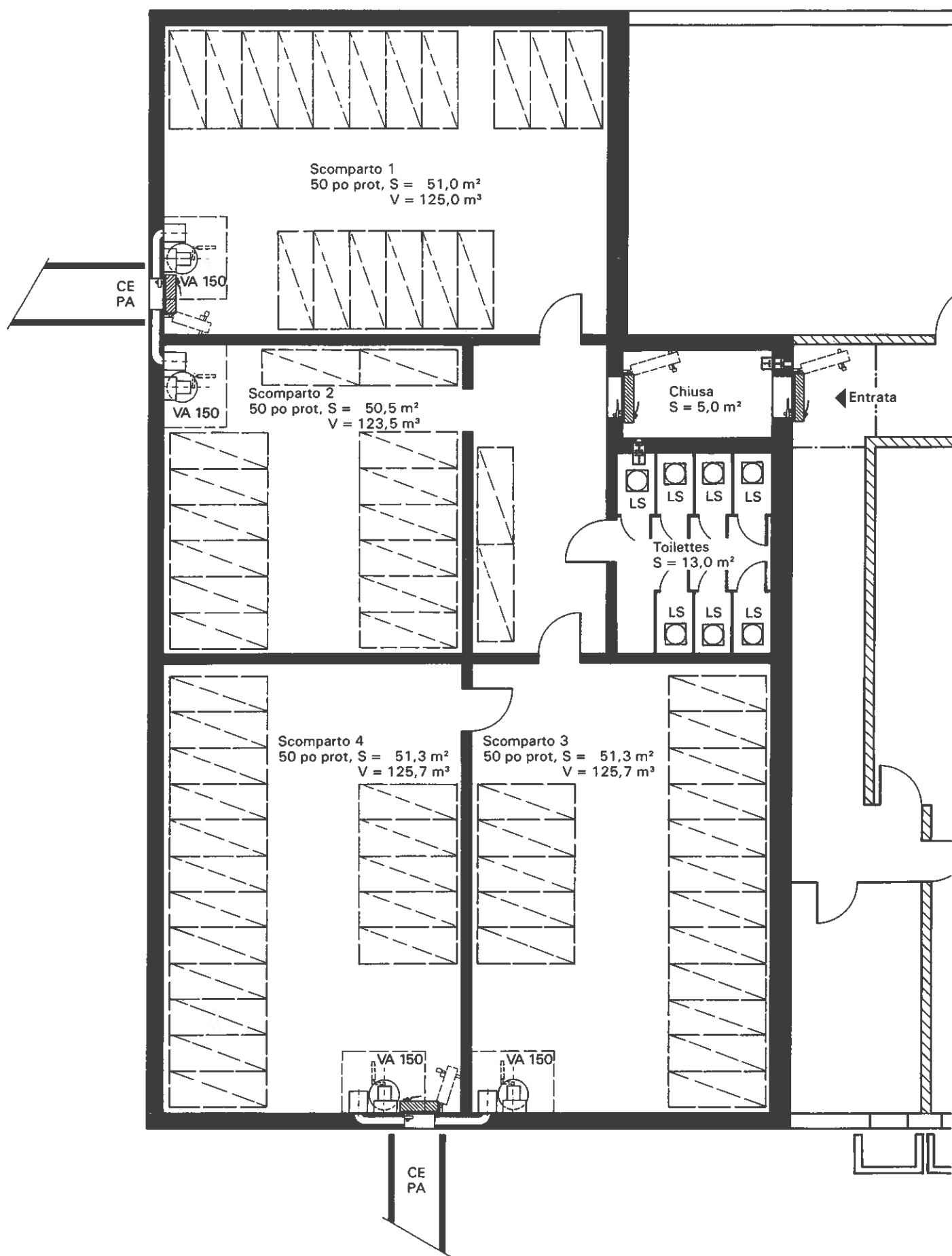
Figura 2.4-14 Rifugio con 200 posti protetti (superficie \geq 217 \text{ m}^2 + 5 \text{ m}^2 )
