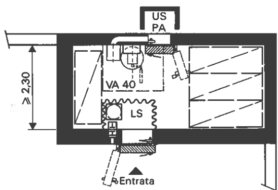
Figura 2.4-5 Pianta per 10 posti protetti (superficie \geq 11 m 2 )
