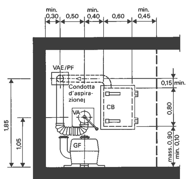
Prospetto Sistemazione con coperchio blindato basso
