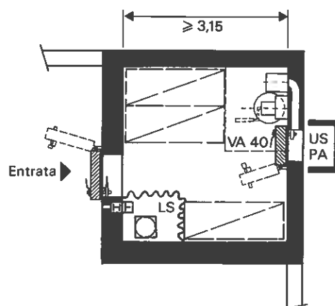
Figura 2.4-4 Pianta per 9 posti protetti (superficie \geq 10 m 2 )
