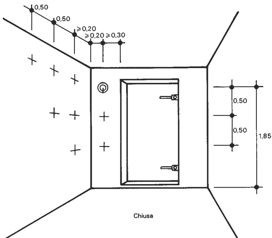
Figura 3.1-2 Disposizione di VSP/VAE nelle pareti delle chiusure
