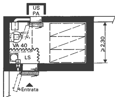
Figura 2.4-3 Pianta per 8 posti protetti (superficie \geq 9 m 2 )
