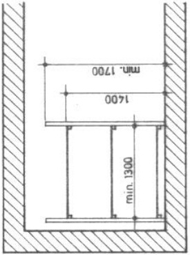
Sezione B di un'unità di 6 posti-letto
