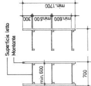
Unità di 3 posti-letto con unità aggiuntiva, disposizione in parallelo
