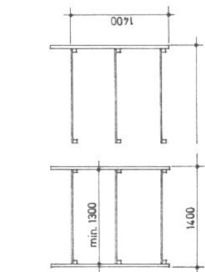
Unità di 6 posti-letto con unità aggiuntiva
