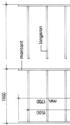
élément de base avec élément additionnel (lits en enfilade)
