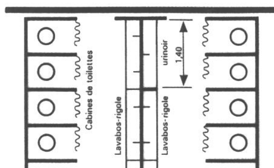
Exemple d'un local de toilettes avec urinoir (plan)
