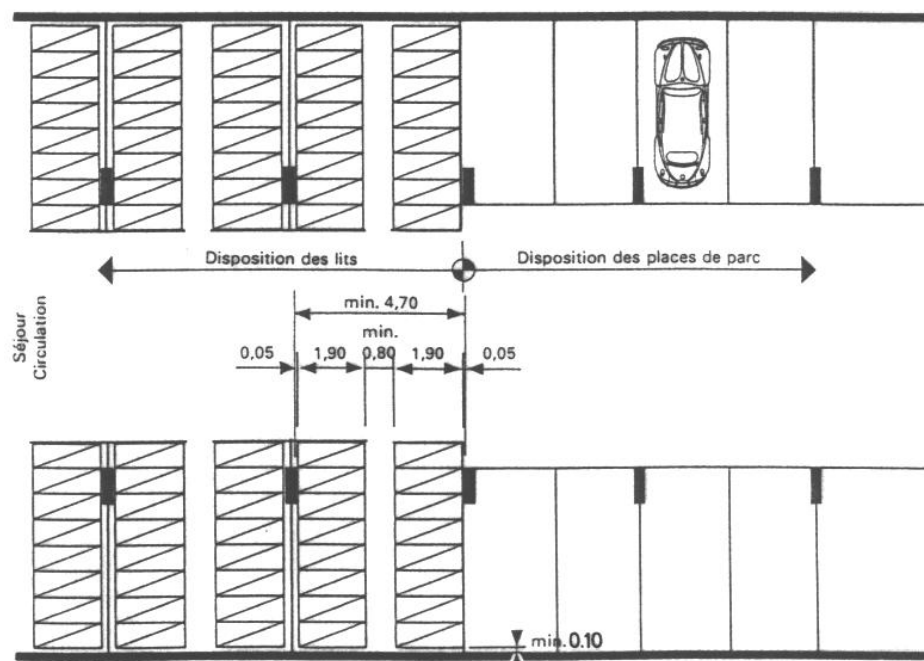
Disposition possible des lits le long des murs, entraxe des piliers env. 5 m
