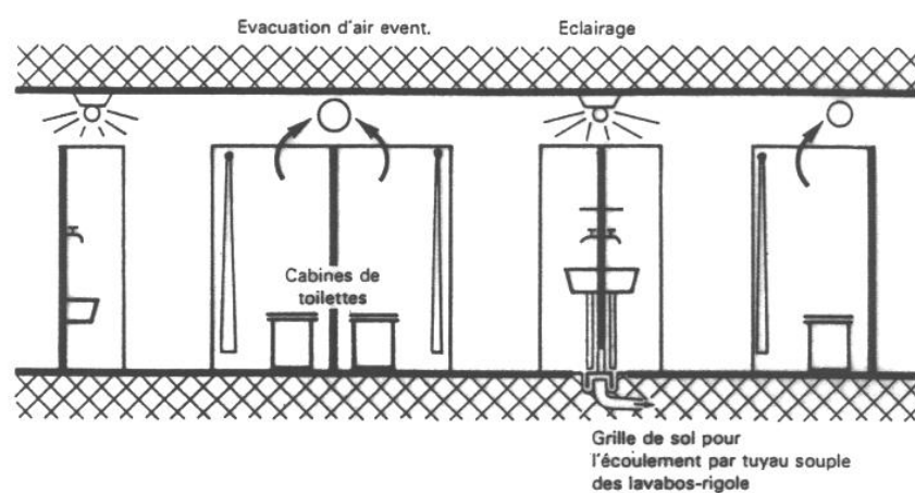
Exemple d'un local de toilettes pour env. 500 places protégées (plan et coupe)
