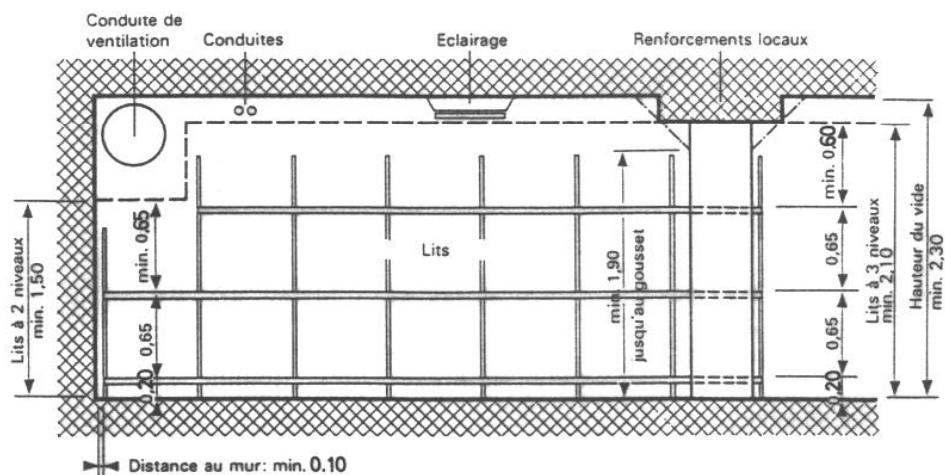
Coupe sur dortoir et réfectoire
