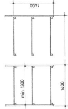
élément de base à 6 lits avec élément additionnel
