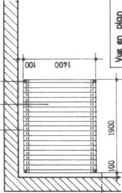
Vue en plan élément de 6 lits
