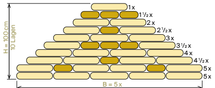
Abb. 45: Aufbau eines Regeldammes mit 5er-Basis (THW)
