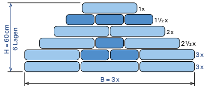
Abb. 43: Aufbau eines Regeldammes mit 3er-Basis (THW)
