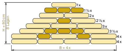
Abb. 44: Aufbau eines Regeldammes mit 4er-Basis (THW)
