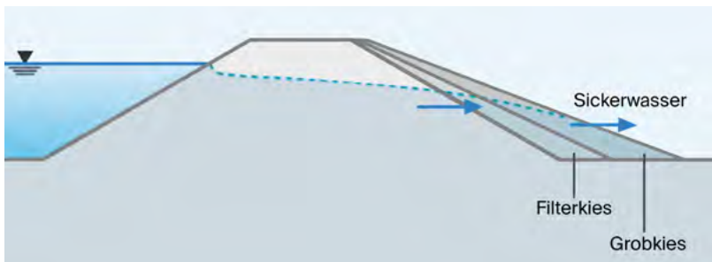
Abb. 75: Stützung eines Damms mit Sandsäcken oder mit Kiesschüttung (Bayerisches Landesamt für Umwelt)
