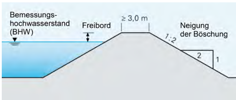
Abb. 69: Geometrie eines Hochwasserschutzdamms (Bayerisches Landesamt für Umwelt)
