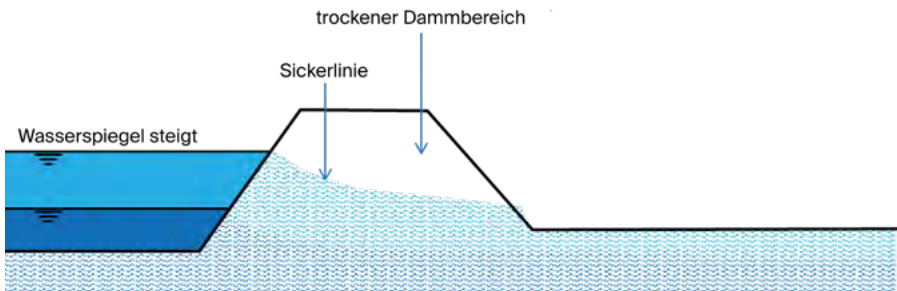
Abb. 70: Sickerlinie am Hochwasserschutzdamm (Bruno Gerber, Tiefbauamt Kanton Bern)
