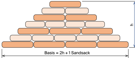
Abb. 42: Aufbau eines normalen Sandsackdammes
