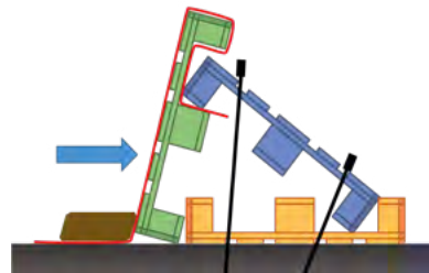
Abb. 57: Konstruktionsprinzip mit drei Paletten (BABS)
