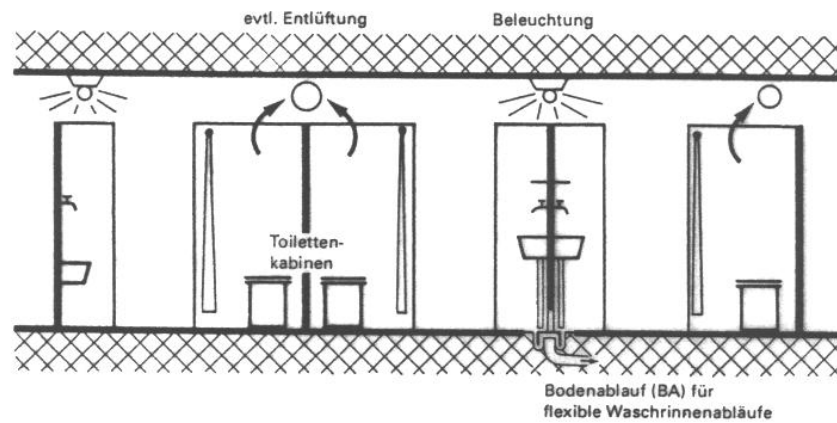
Beispiel eines Toilettenraumes für ca. 500 Schutzplätze (Grundriss und Schnitt)
