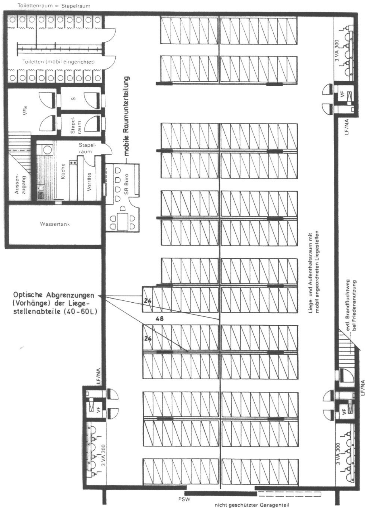
Schutzraum mit rund 600 Schutzplätzen in Tiefgarage (Grundriss)
