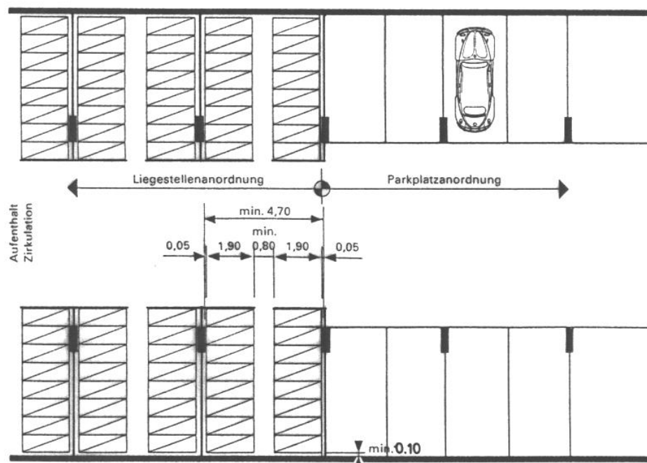
Mögliche Liegestellenanordnung entlang den Wänden, Stützenabstand ca. 5 m
