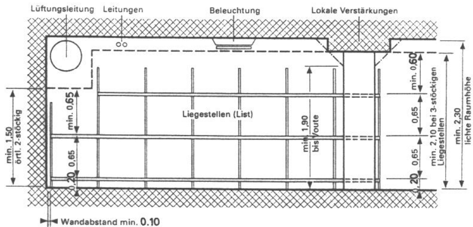
Querschnitt durch Liege- und Aufenthaltsraum
