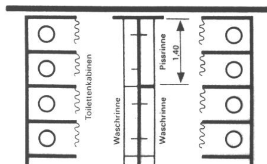
Beispiel Toilettenraum mit Pissrinne (Grundriss)
