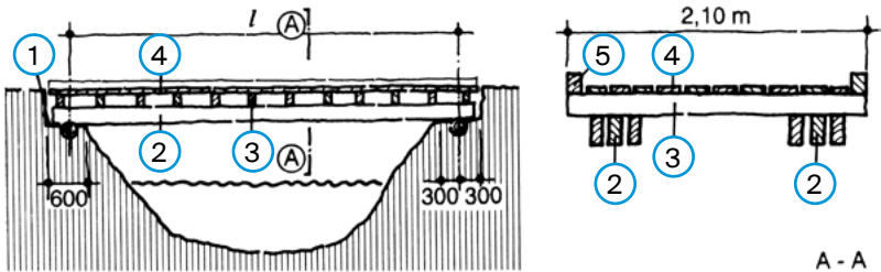
Abb. 78: Notbrücke mit einer Spannweite von l bis zu 6 Metern (Schweizer Armee)
