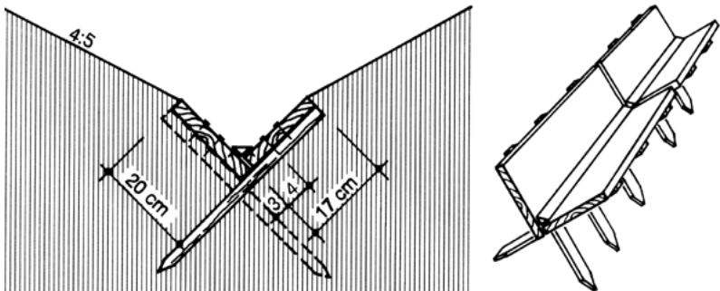
Abb. 50: Dreieckskännel (ASTRA)
