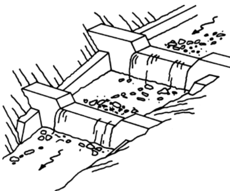
Abb. 53: Bestandteile einer Wildbachverbauung – Holzkasten und einwandige Holzsperrn (ASTRA)
