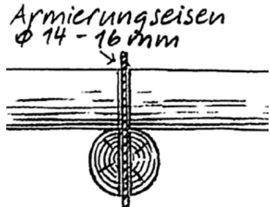
Abb. 45: Kreuzungsstelle (ASTRA)
