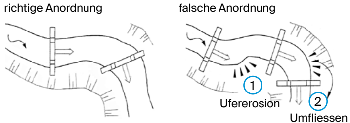
Abb. 54: Querwerke im Grundriss
