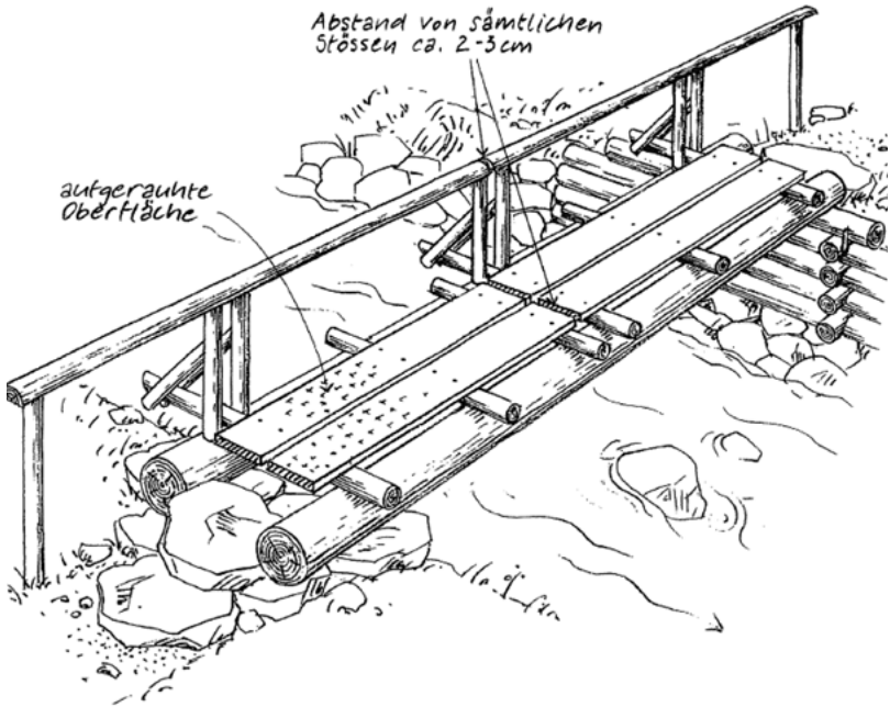
Abb. 79: Rundholzbrücke (ASTRA)
