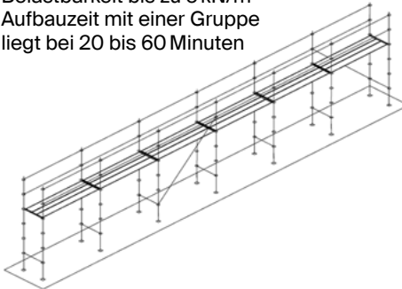
Abb. 96: Skizze Hochwasserlaufsteg mit Gerüstmaterial (THW)
