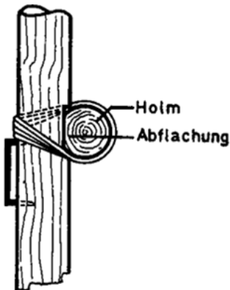
Abb. 92: Sicherung und Verbindung Holm mit Bockfuss
