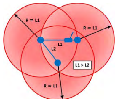
Abb. 32: Schleuderbereich bei einem umgelenkten Seilzug
