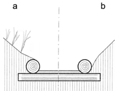
Abb. 52: Einbettung a richtige Ausführung - b falsche Ausführung (ASTRA)
