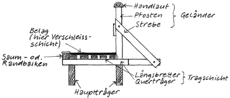
Abb.75: Brückenbauteile (Astra)
