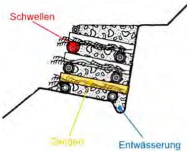
Abb. 44: Skizze doppelwandiger (doppelter) Holzkasten (ASTRA)
