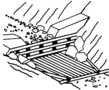
Abb.61: Fallboden aus Holz
