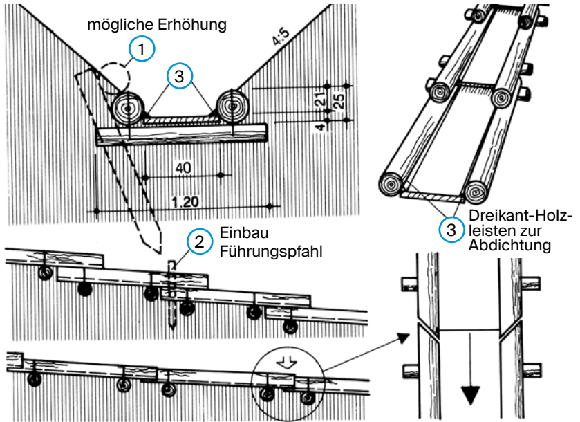
Abb. 51: Rundholz-Rechteckkännel (ASTRA)
