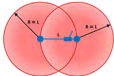
Abb. 31: Schleuderbereich bei direktem Seilzug
