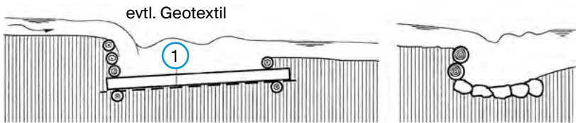
Abb. 64: Kolkenschutz (Holzrost, links; Blöcke, rechts)
