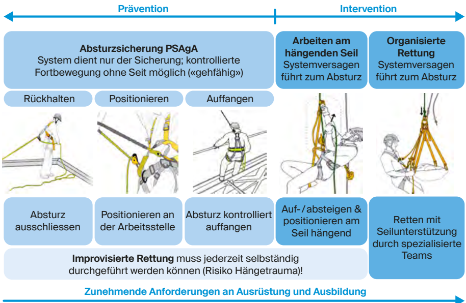
Abb.1: Systematik und Abgrenzung der Absturzsicherung (BABS)
