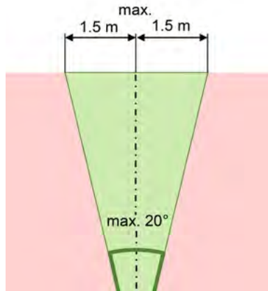
Abb. 34: Faustregel zulässige Arbeitszone an der Absturzkante (Grundriss) (BABS)
