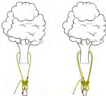
Abb. 48: Ein-Punkt-Verankerung (SFV)
