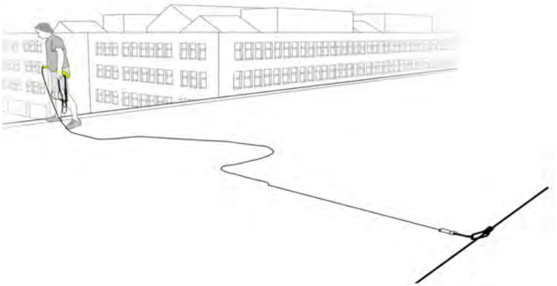
Abb. 35: Gefahr Schlaffseil (Petzl)
