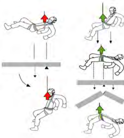
Abb. 9: Unterschiede beim Sturz in eine Auffangöse oder in eine Hüftöse (ventrale Halteöse) (Petz)
