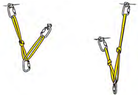
Abb. 57: Ein- oder zweiseitiges Abknoten der Verbindungen bei einer Ausgleichsverankerung (Petzl)
