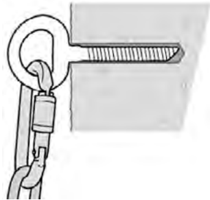
Abb. 50: Klebanker (Petzl)
