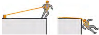
Abb.23: Grenzen beim Rückhalten (Petzl)
