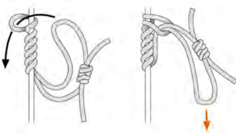
Abb. 43: Kreuzklemmknoten (SAC)
