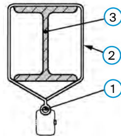
Abb. 44: Anschlagssystem gemäß EN 795 (EN-Normen)
