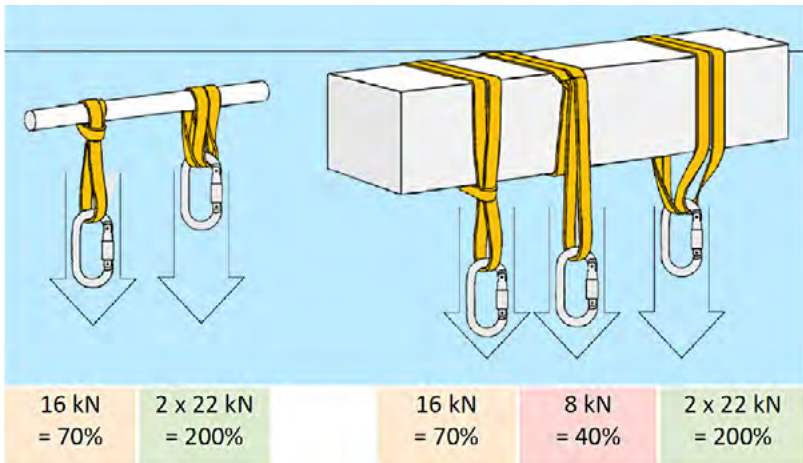
Abb. 46: Auswirkungen verschiedener Anschlagarten mit einer Bandschlinge EN 795 (MBL = 22 kN) auf die Endfestigkeit des Anschlagpunktes (Gantner/Merk)
