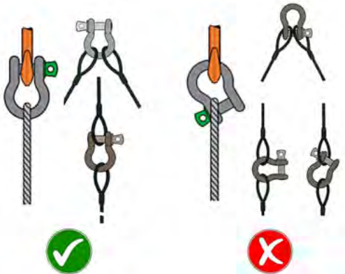
Abb.26: Richtige Anwendung von Schäkeln (Kloska Group)
