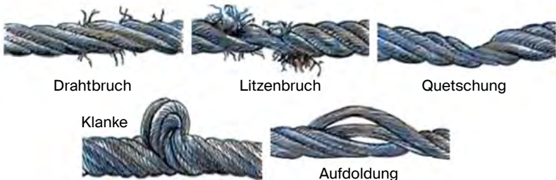
Abb. 29: Mögliche Arten der Beschädigung an Drahtseilen (Berufsgenossenschaft der Bauwirtschaft)
