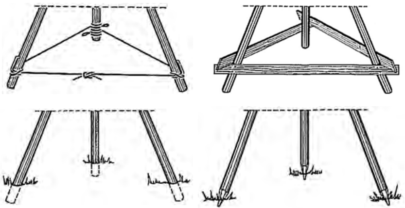
Abb. 43: Methoden zum Sichern der Beine gegen Wegrutschen (THW).
