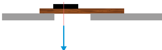
Abb. 21: Anschlagen des Verbindungsmittels bei breiten Öffnungen, mit Querriegel und Verstärkungsholz (Grundriss)
