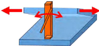
Abb. 63: Horizontale Kraft bei angewinkeltem Hebeegerät
