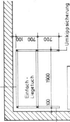
Grundriss 3er - Einheit
